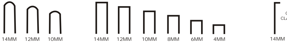
GRAPAS CUADRADA Y REDONDA
